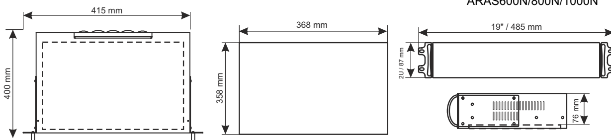
Montaż na szynie ARAS600N/800N/1000N
