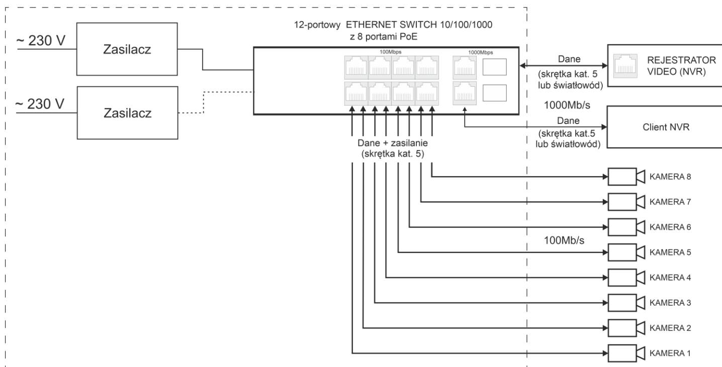
Rys. 1. Schemat blokowy.
